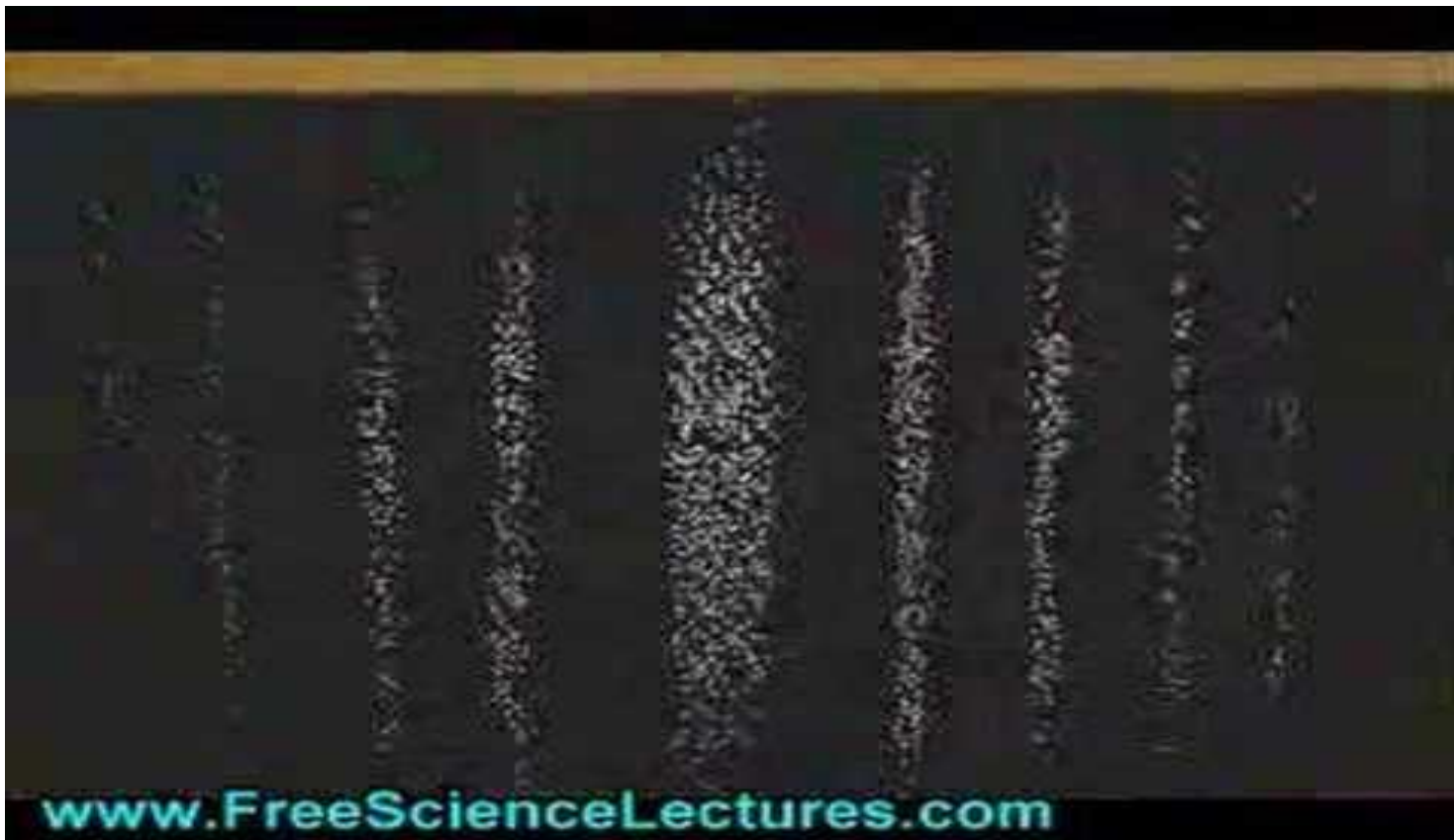
ACTUAL PARTICLE INTERFERENCE PATTERN
